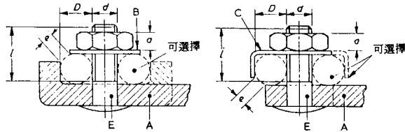
需用墊圈或夾片的螺絲
