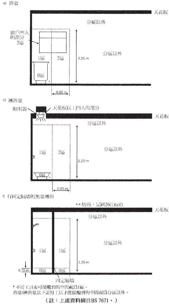
分區尺寸的例子(剖面圖)
