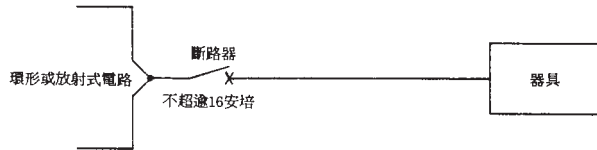
(B) 斷路器保護
