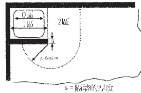
f) 有固定隔牆的無盆淋浴
