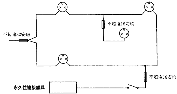
(A) 環形電路
