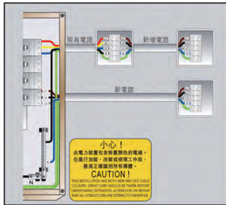
圖 A18(6) - 加裝、改裝或修理現有三相裝置
