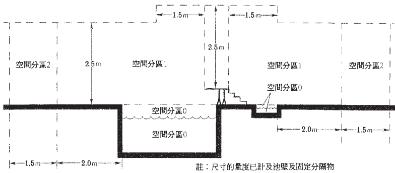
泳池及鱗水池的分區尺寸
