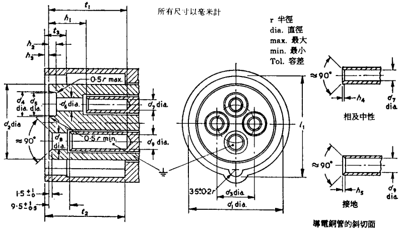
導電銅管的斜切面
