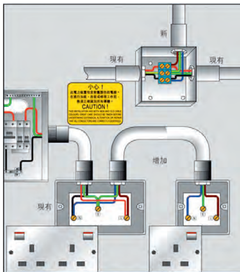
圖 A18(4) - 在現有單相裝置進行加裝、改裝或修理工作(現有相線以紅色識別)
