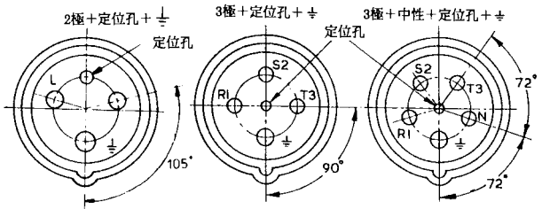
導電銅管的排列及終端標誌 插座或連接器導電銅管的正視圖
