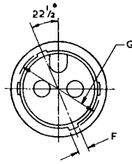
插座的正視圖
