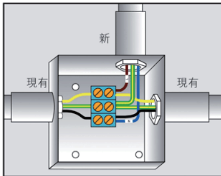
圖 A18(5b) - 加裝、改裝或修理現有單相裝置 (現有相線以黃色識別)
