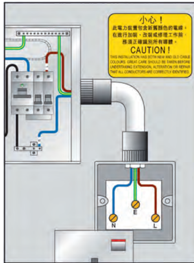
圖 A18(5c) - 在現有配電箱加裝新顏色代碼電線 (現有相線以藍色識別)
