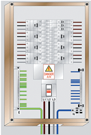
圖 A18(2b) - 三相配電箱內的新顏色代碼電線
