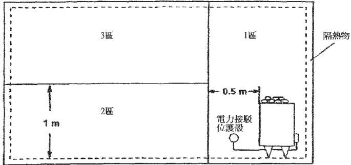
蒸汽浴室的分區尺寸
