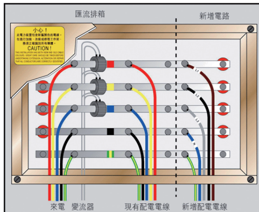
圖 A18(7) - 現有三相裝置的匯流排箱的新舊顏色代碼電線接駁處
