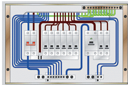
圖 A18(2a) - 單相配電箱內的新顏色代碼電線
