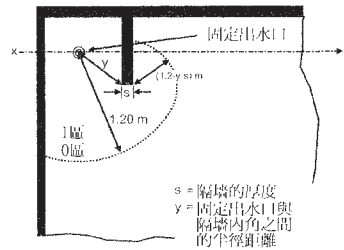
f) 有固定隔牆的無盆淋浴
