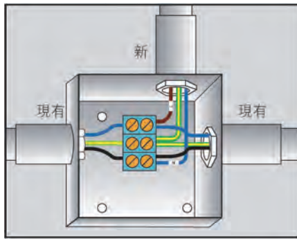
圖 A18(5d) - 加裝、改裝或修理現有單相裝置 (現有相線以藍色識別)
