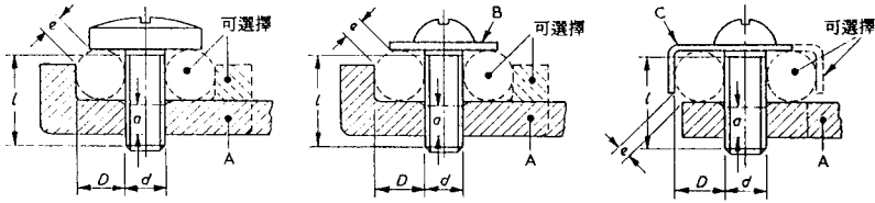
不需用墊圈或夾片的螺絲
