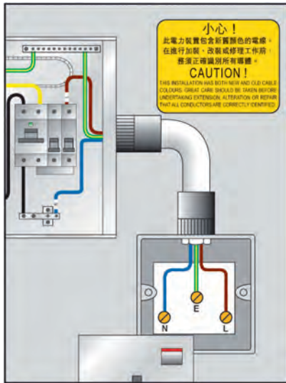
圖 A18(5a) - 在現有配電箱加裝新顏色代碼電線 (現有相線以黃色識別)
