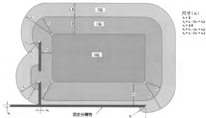
有最少2.5m高固定分隔物的分區尺寸(平面圖)的例子
