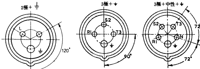
導電銅管的排列及終端標註 插座或連接器導電銅管的正視圖
