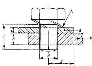
A 鎖定設備 B 電纜線耳或片
