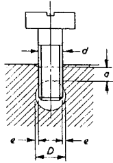
無壓片的終端
