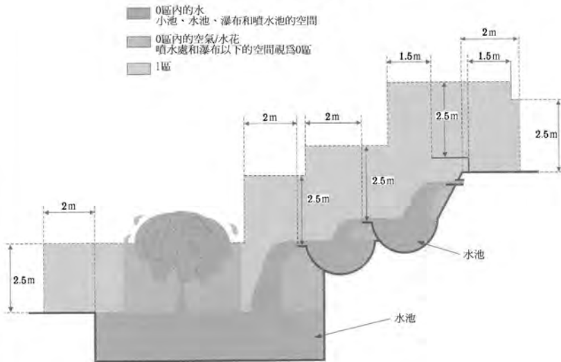
如何界定噴水池分區的例子
