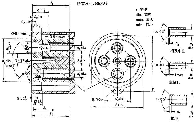
導電銅管的斜切面
