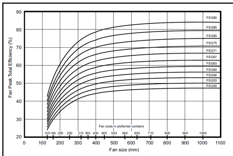
Figure 6.15 (b) : Fan Efficiency Grade (FEG)
