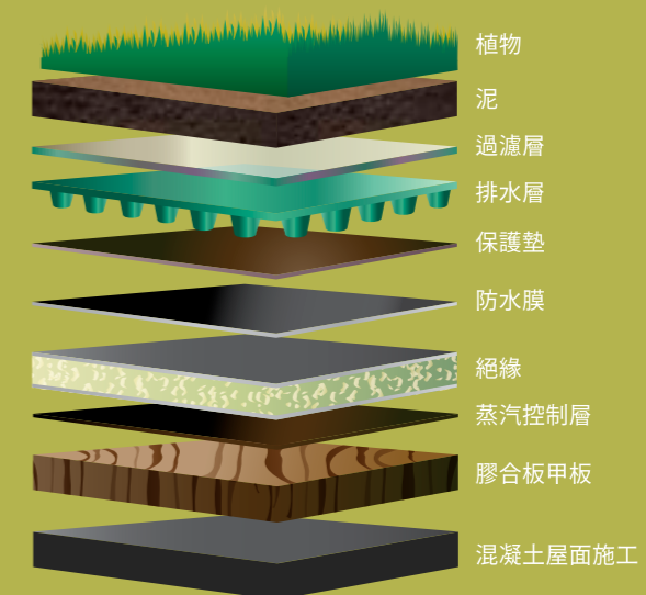
屋頂綠化的典型結構
