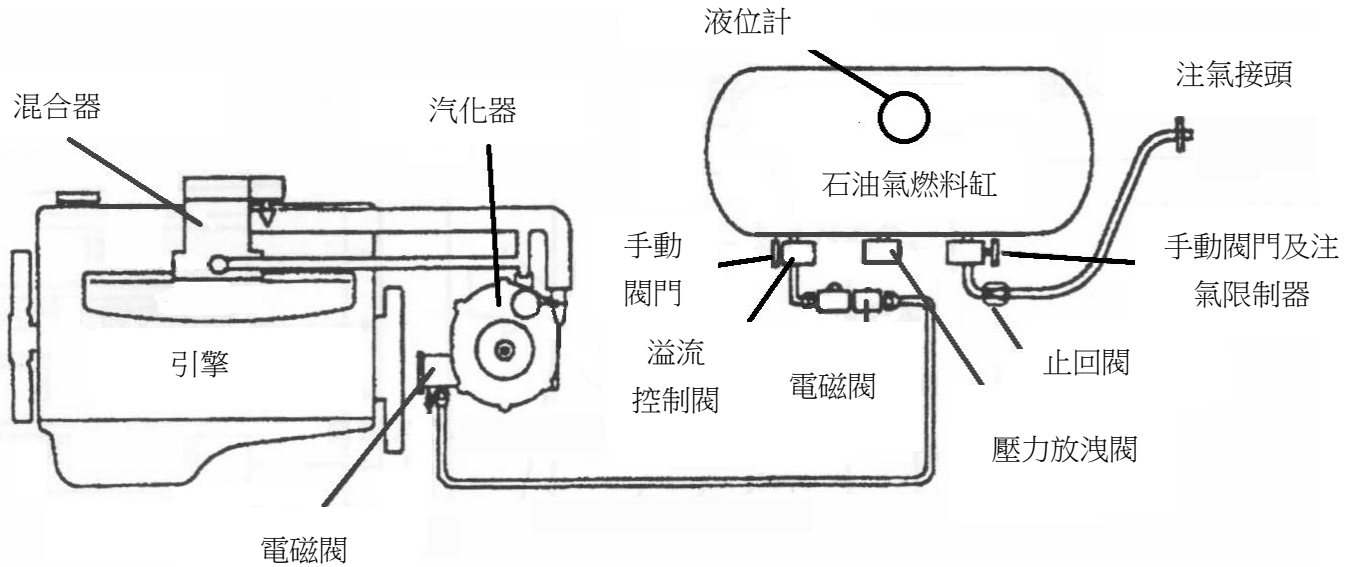
圖A1：燃料汽化系統
