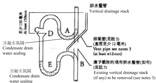
iii) 排水管的其他設計方法 Alternative design at vertical draining stack
