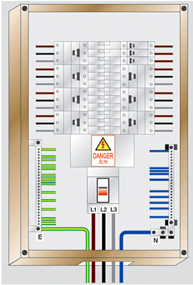
圖 A18(2b) - 三相配電箱內的新顏色電線
