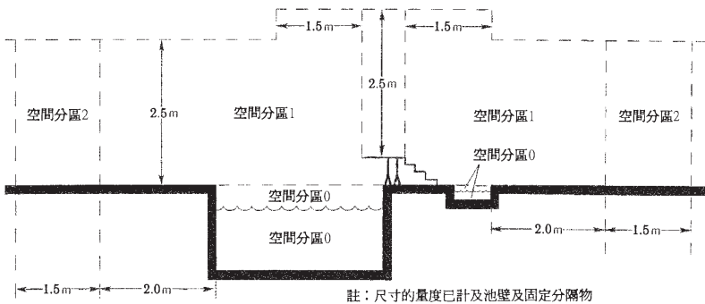
泳池及嬉水池的分區尺寸
