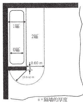
b) 有固定隔牆的浴盆
