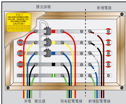
圖 A18(7) - 現有三相裝置的匯流排箱的新舊顏色電線接駁處
