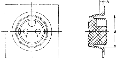
插座
