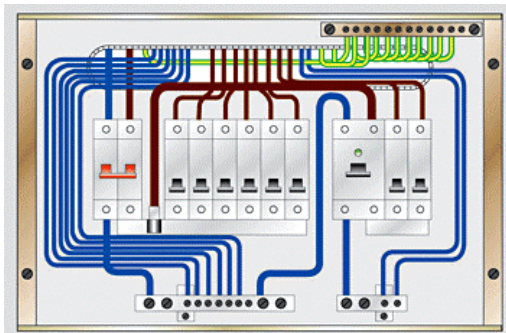
圖 A18(2a) - 單相配電箱內的新顏色電線
