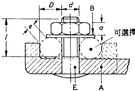
螺旋式終端
