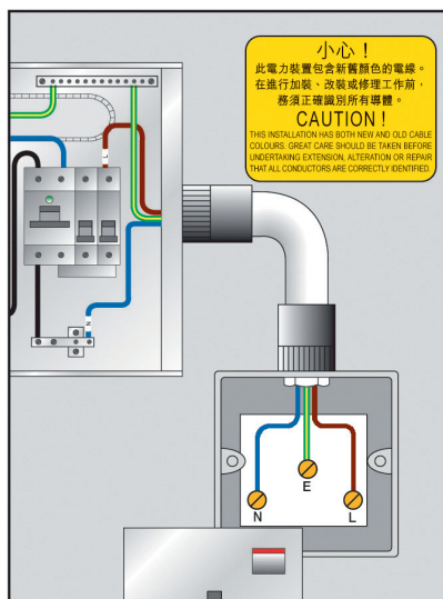
圖 A18(5c) - 在現有配電箱加裝新顏色電線 (現有相線以藍色識別)
