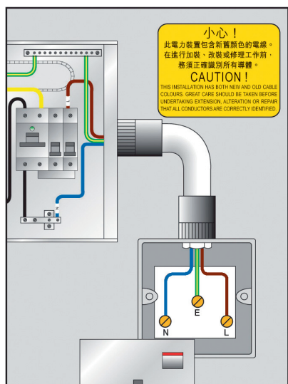
圖 A18(5a) - 在現有配電箱加裝新顏色電線 (現有相線以黃色識別)
