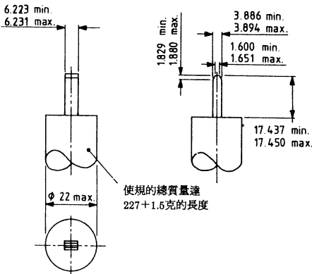
(b) 相線及中性線載流插座觸點規
