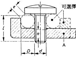
不需用墊圈或夾片的螺絲
