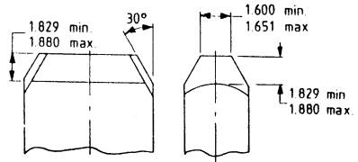
(c) 接地插座觸點規60° 錐面的部分
