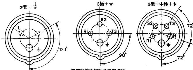
導電銅管的排列及終端標誌 插座或連接器導電銅管的正視圖
