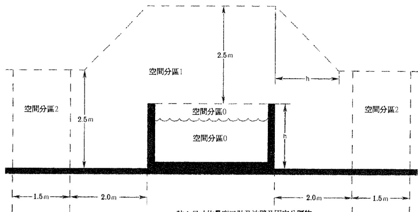
高於地面水平的水池的分區尺寸
