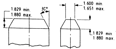
(d) 接地插座觸點規的削角 (相線及中性線 插座觸點規只在較長一邊削角)
