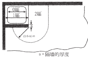
f) 有固定隔牆的無盆淋浴
