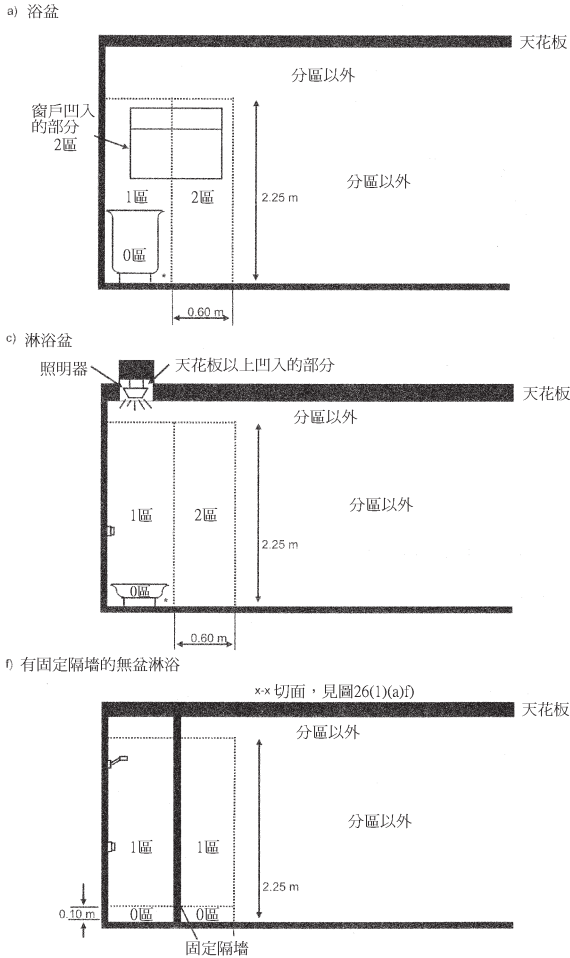
分區尺寸的例子(剖面圖)
