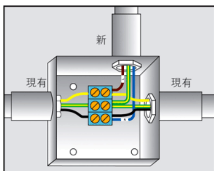
圖 A18(5b) - 加裝、改裝或修理現有單相裝置 (現有相線以黃色識別)
