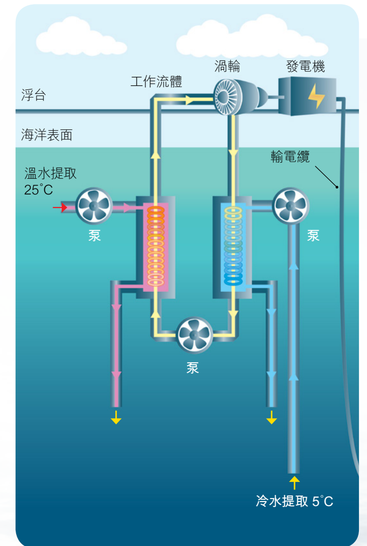
海洋熱能轉換示意圖
