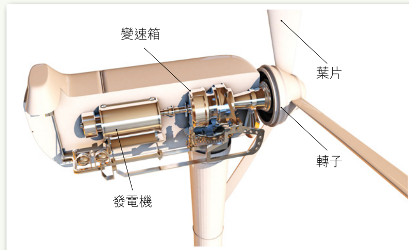
風力發電機內部組件
