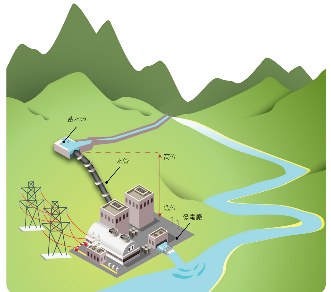
徑流式水電站
