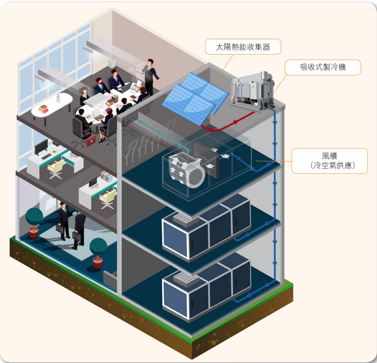
太陽能製冷系統
