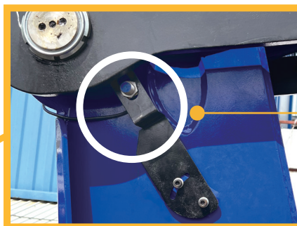
可探测吊臂位置的 传感器
