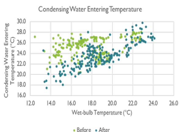
图 A.6(c)冷凝器进水温度与湿球温度对比
