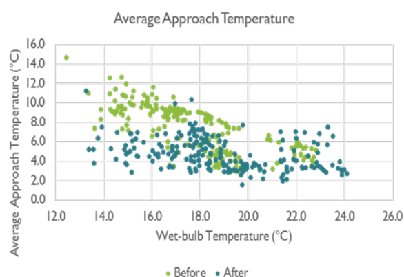
图 A.6(b)平均趋近温度(approach temperature)与湿球温度对比
