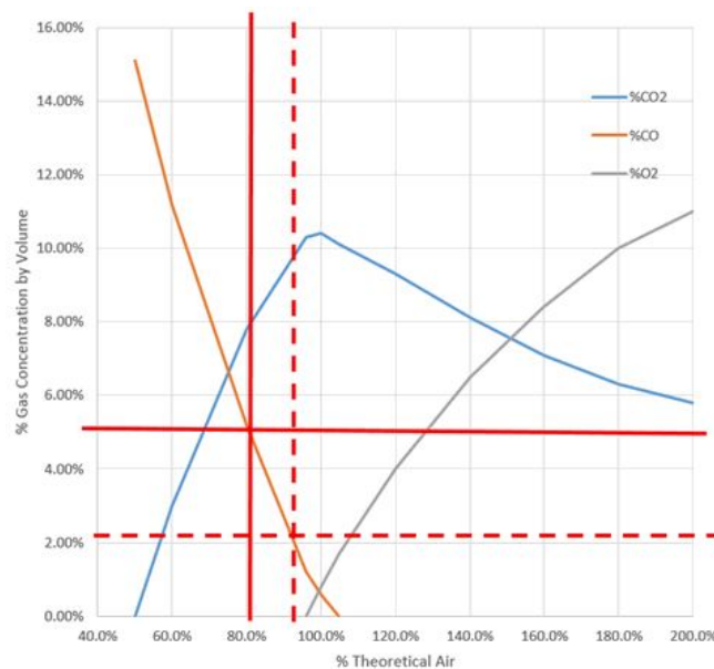
圈 A.15(b)理论燃烧
