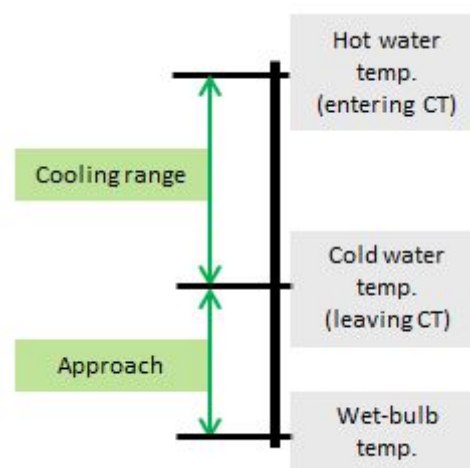
图 A.6(b)平均趋近温度(approach temperature)与湿球温度对比
