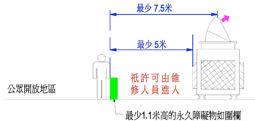
圖B5 — 設置永久而固定的障礙物
