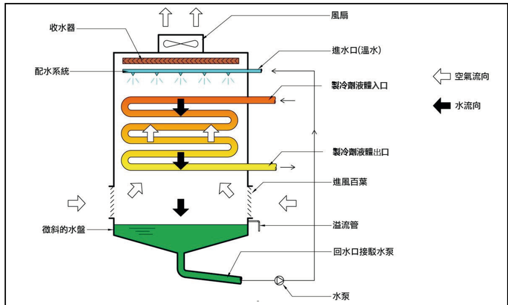
圖1.9：蒸發式冷凝器的典型配置
