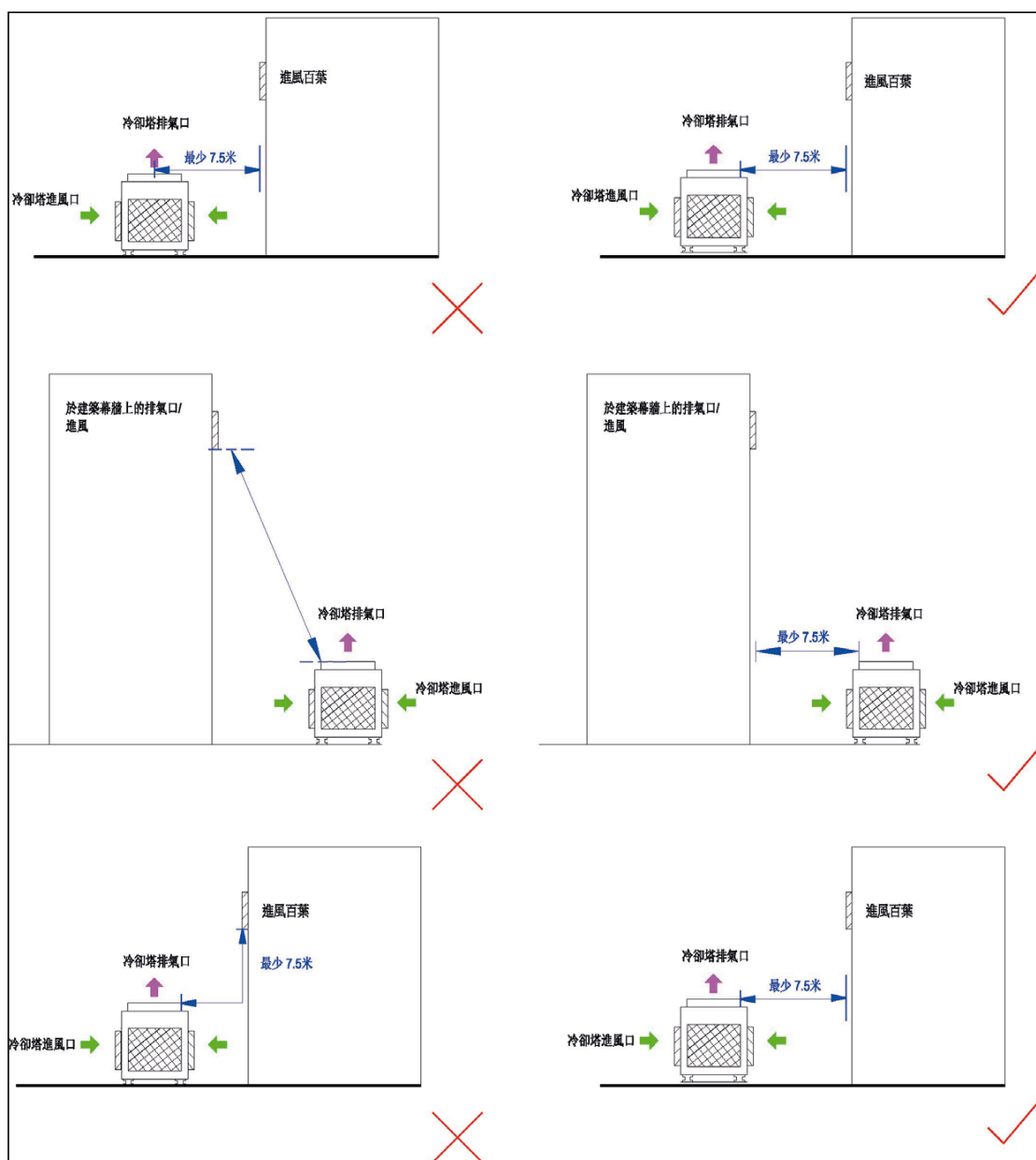
圖B1 — 一般距離的量度方法
