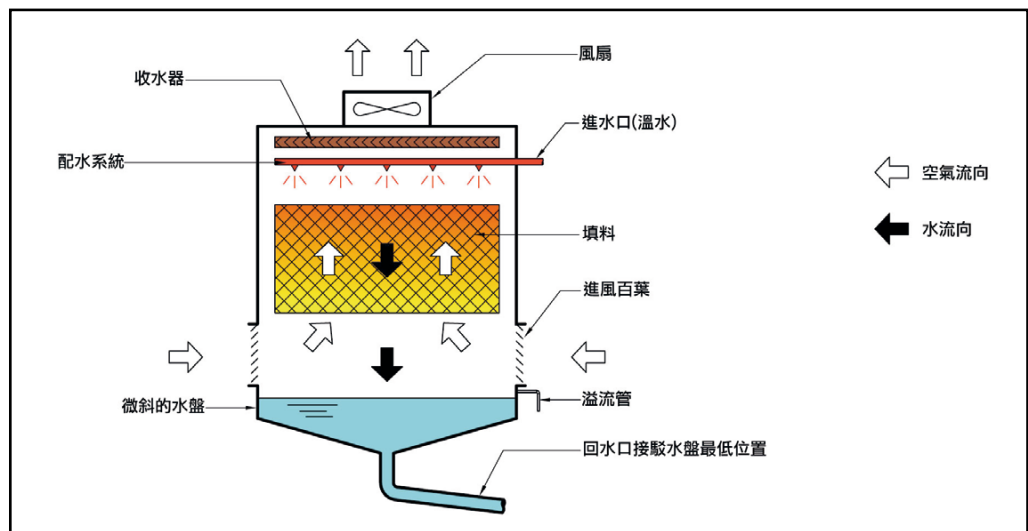
圖1.3：引風逆流式冷卻塔的典型配置
