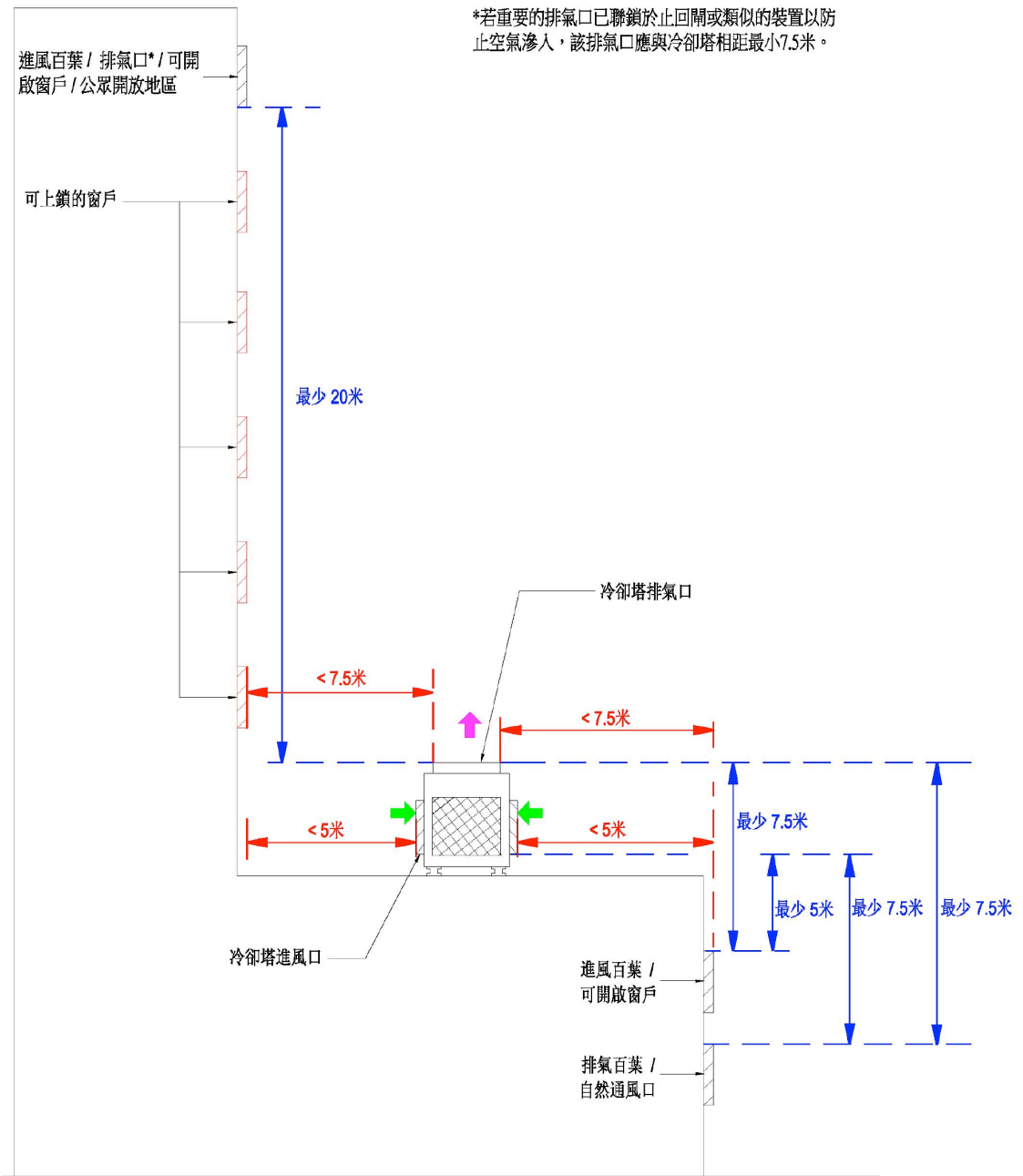
圖B3 — 垂直分隔距離
