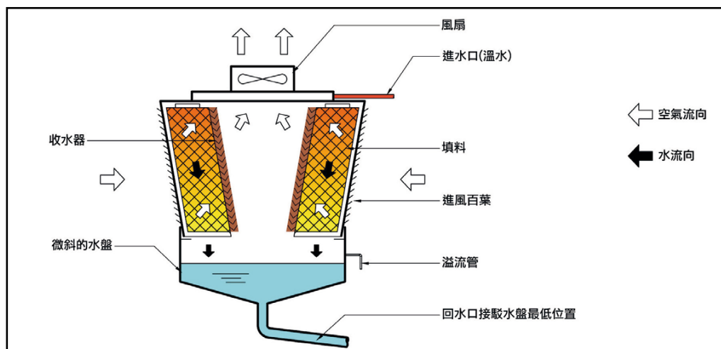
圖1.4：引風橫流式冷卻塔的典型配置
