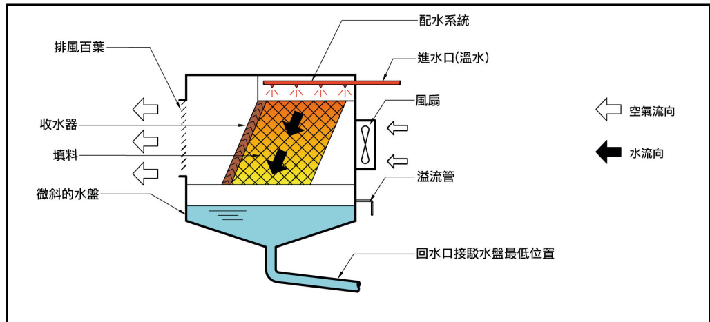
圖1.6：鼓風橫流式冷卻塔的典型配置
