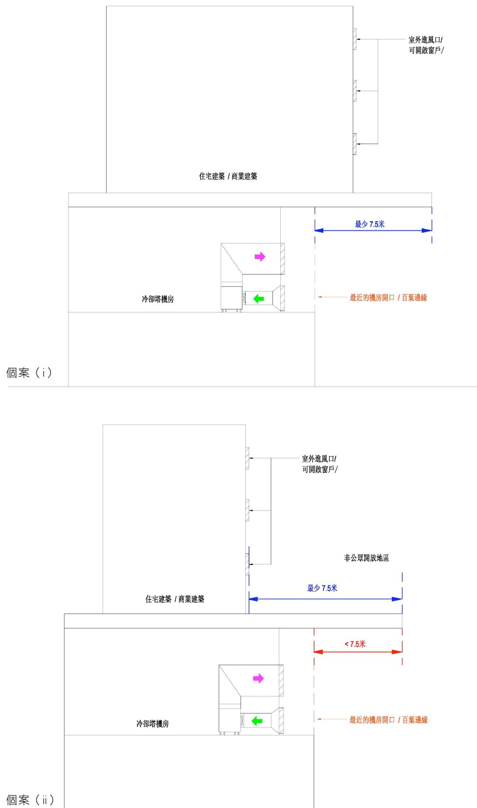
圖 B10 - 裝置於延伸平台下的冷卻塔
