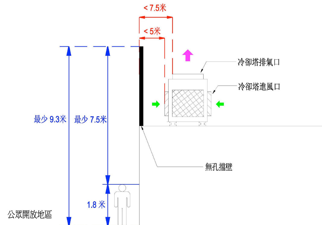
圖 B7 — 設置無孔擋壁
