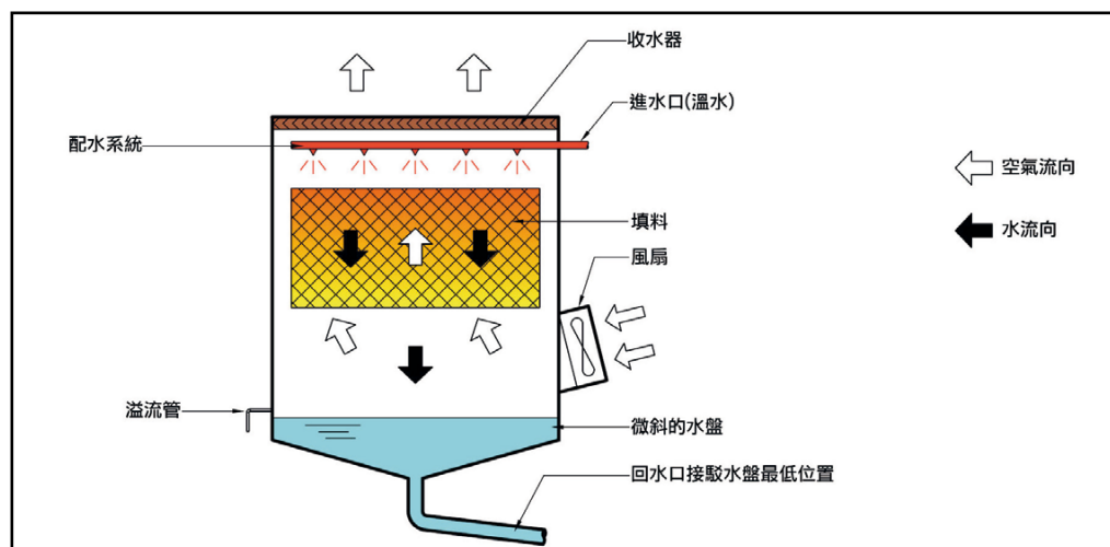
圖1.5：鼓風逆流式冷卻塔的典型配置
