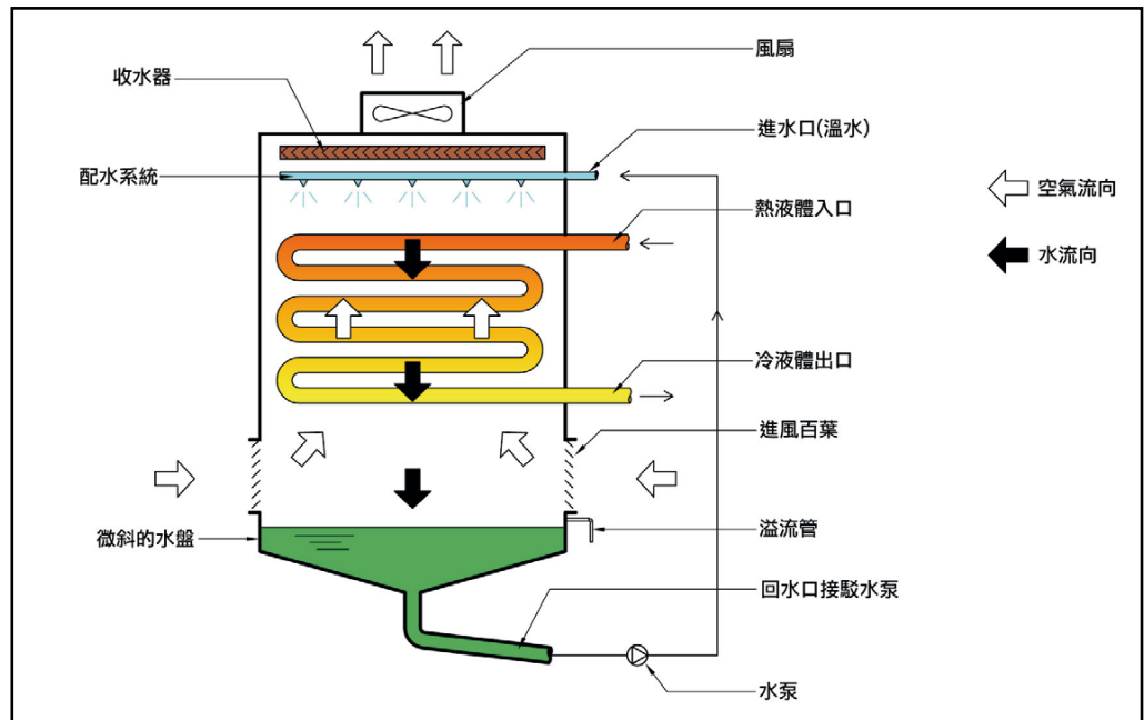
圖1.7：沒有填料的密閉式冷卻塔的典型配置
