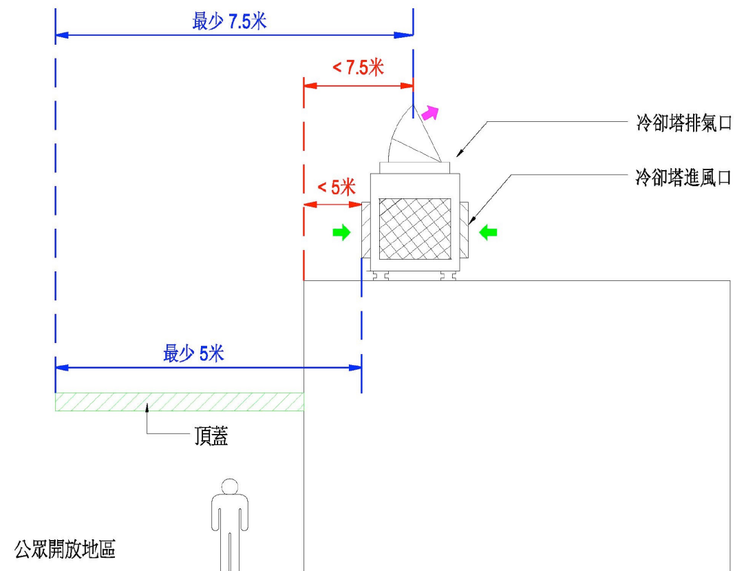
圖B6 — 設置頂蓋
