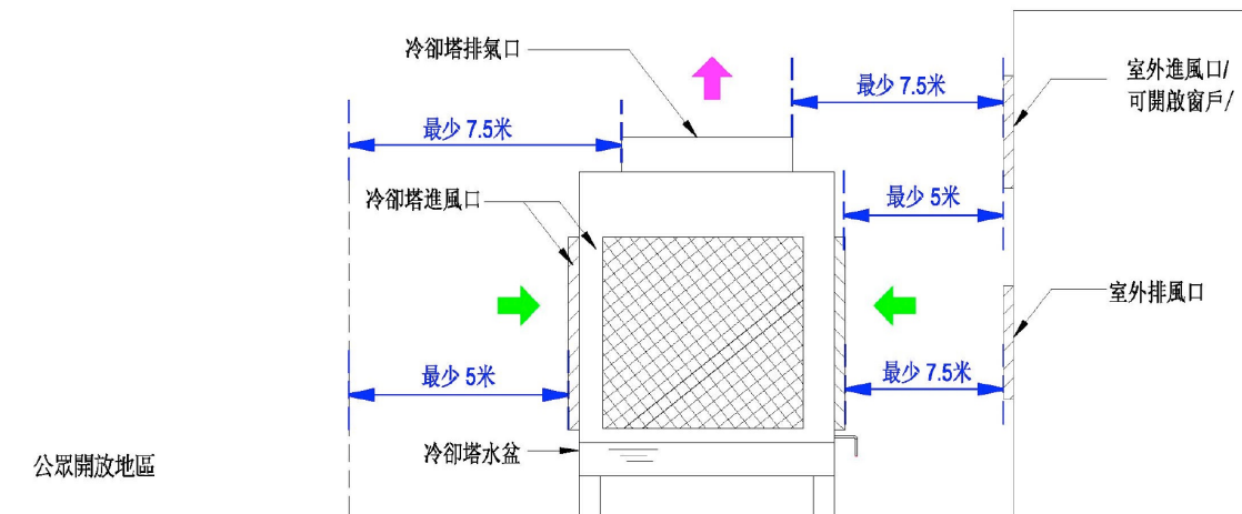
圖B2 — 一般距離的量度
