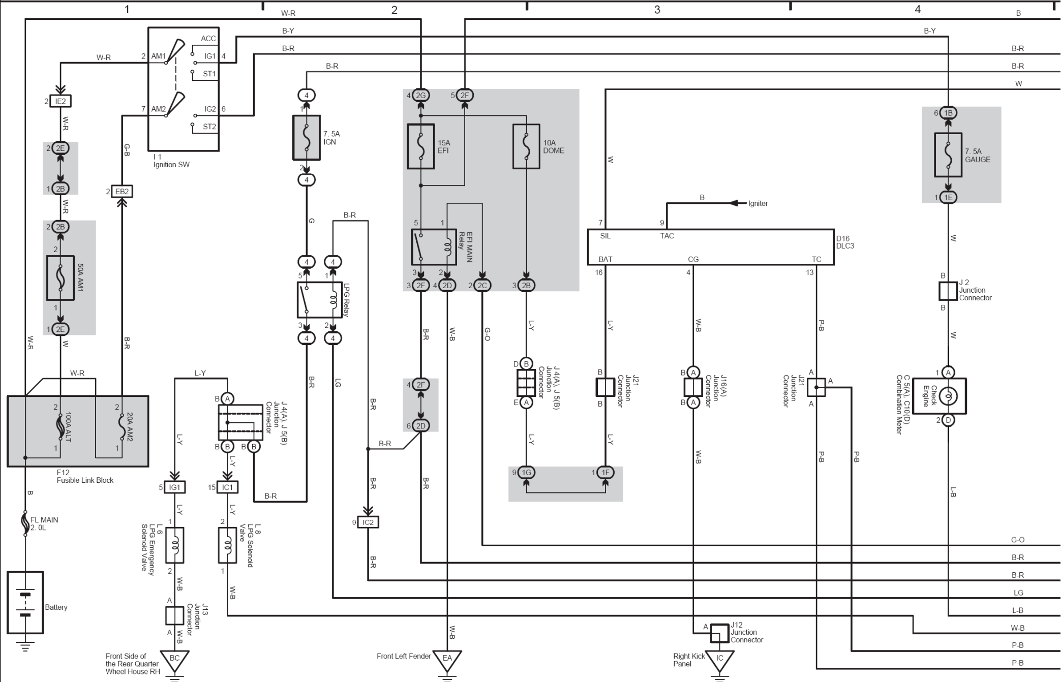
豐田五座位石油氣引擎控制電路圖
