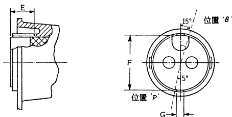
插座正面的正視圖
