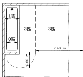
b) 有固定隔牆的浴盆
