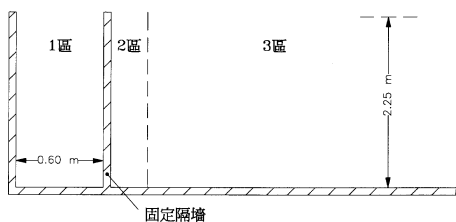
i) 有固定隔牆的無盆淋浴
