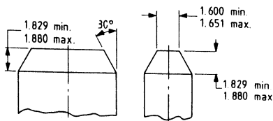
(d) 接地插座觸點規的削角 (相線及中性線 插座觸點規只在較長一邊削角)
