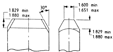
(c) 接地插座觸點規60° 錐面的部分
