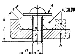
螺旋式終端
