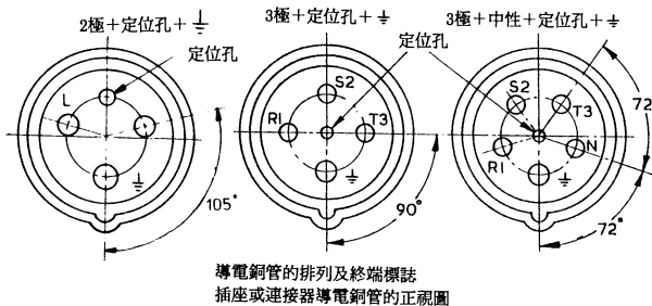
63安培及125安培有鎖扣器件插座的尺寸及觸點構形
