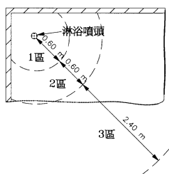
e) 無盆淋浴
