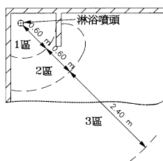
f) 有固定隔牆的無盆淋浴
