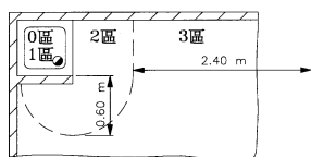
d) 有固定隔牆的淋浴盆
