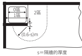
d) 有固定隔牆的淋浴盆
