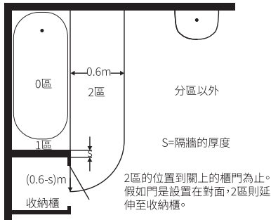
g) 收納櫃旁的浴缸
