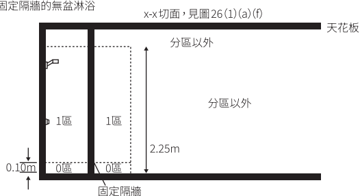
c) 有固定隔牆的無盆淋浴
