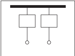
形式2 分隔匯流排和所有功能單元
