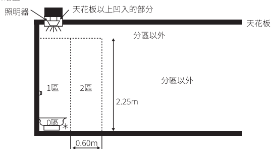
c) 有固定隔牆的無盆淋浴
