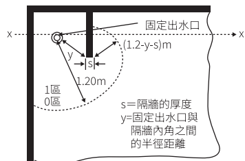
f) 有固定隔牆的無盆淋浴
