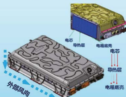
(e) 散熱系統
