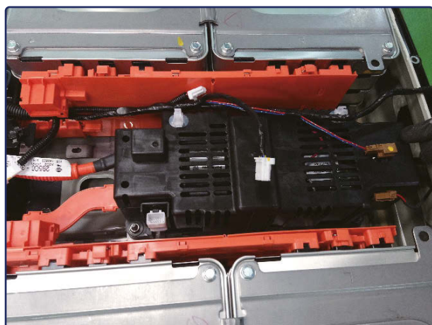
(a) 集電網路及線束
