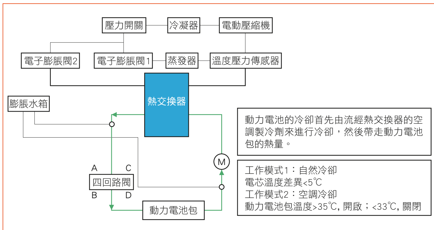
電池冷卻系統工作原理（圖2）
